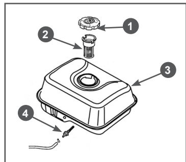
Рис. 18 Топливные фильтры
